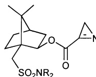
1a ; R = Et 1b ; R = Cyclohexyl
